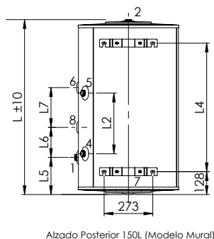
Alzado Posterior 150L (Modelo Mural)
